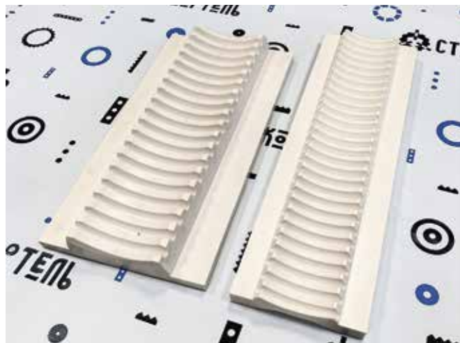
Рис. 6. Комплект реек перемещения стола и шпиндельной бабки для горизонтально-расточного станка модели 2H637GF1. Материал – ZEDEX ZX-100K
