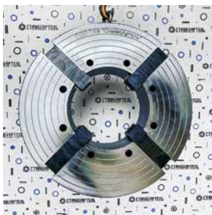
Рис. 3. Патрон \varnothing 720 мм станков 1Н983, 1А983, СА983, РТ783
